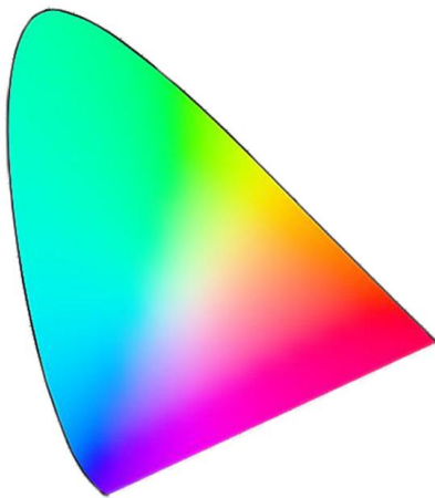
“Commission Internationale de l’Éclairage” (CIE) Colour Diagram
